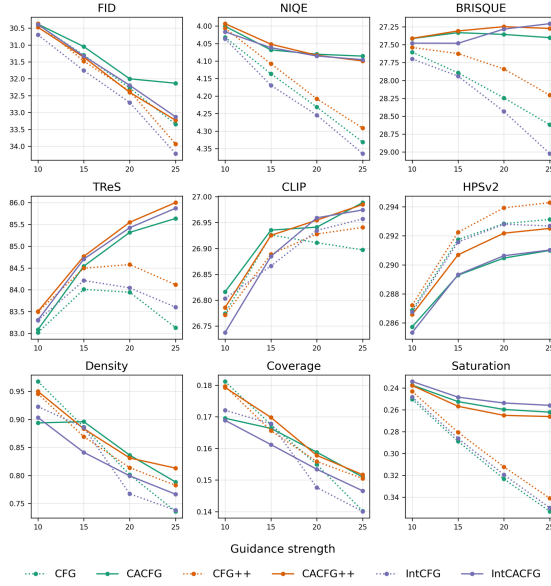
(b) COCO
