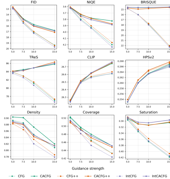
(b) COCO
