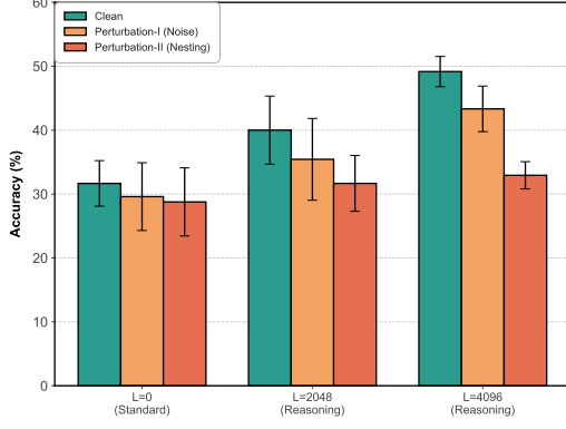
(a) Qwen3-14B
