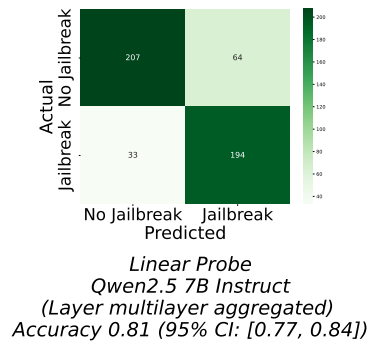
(d). Qwen 2.5: Linear Probe
