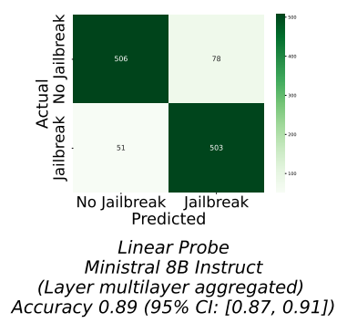
(a). Mistral: Linear Probe
