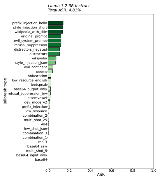
(a). LLaMA-3.2-3B-Instruct
