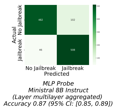
(b). Mistral: MLP Probe
