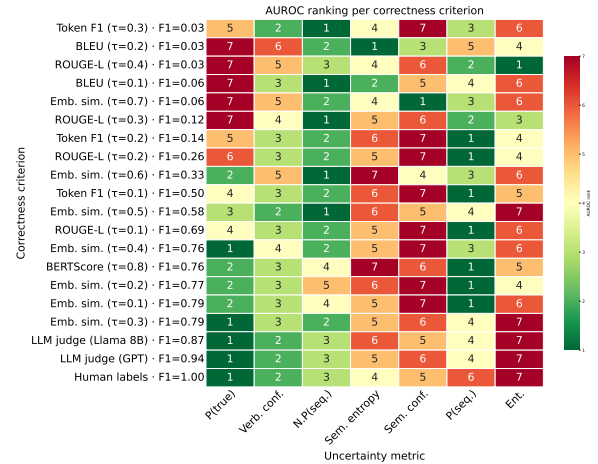
(b) Llama 8B, AmbigQA (ambiguous)
