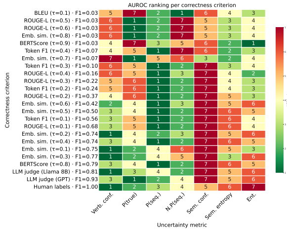
(a) Llama 3B, AmbigQA (ambiguous)
